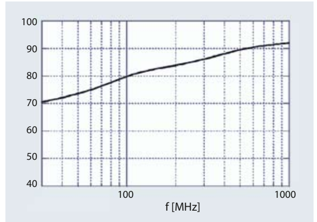
Schirmdämpfung von Dübelplatten, vermessen nach IEEE Std. 299
